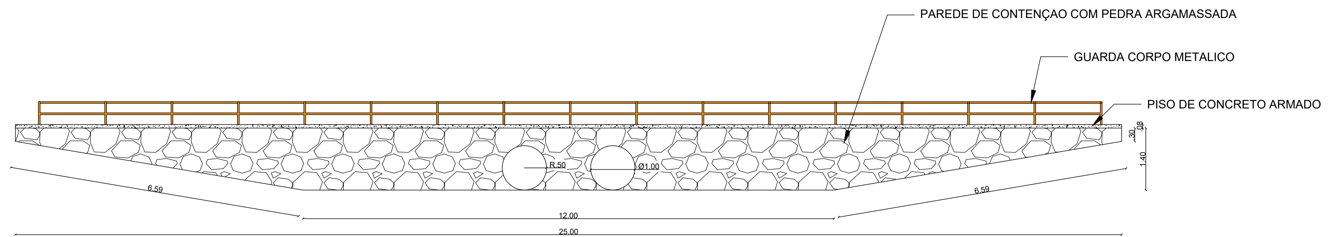
1 CORTE AA ESCALA — 1 : 50
