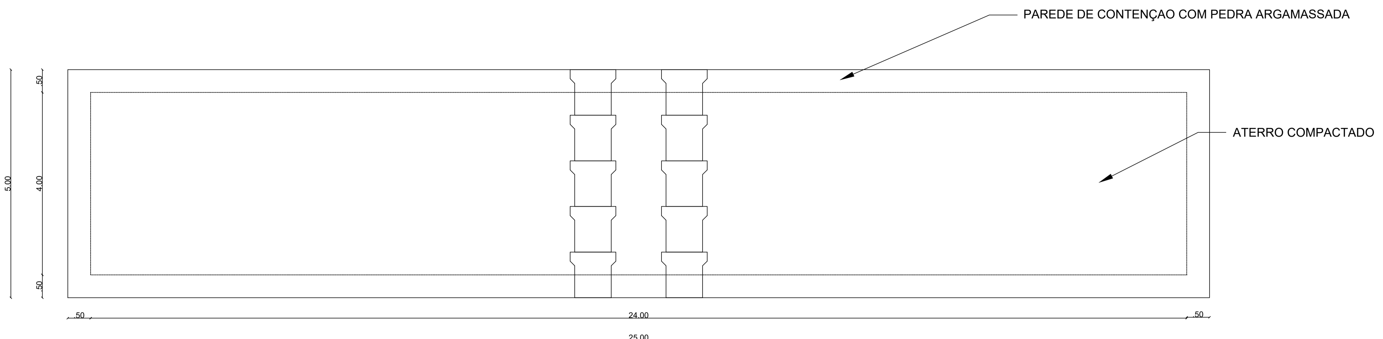
1 PLANTA BAIXA - PASSAGEM MOLHADA ESCALA — 1 : 50
